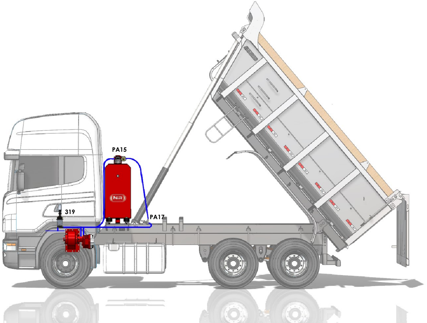
319 - VÁLVULA NEUMÁTICA MONOCOMANDO 1/8" BSP no incluida en el kit
